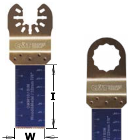
OMM10 Universalaufnahme
