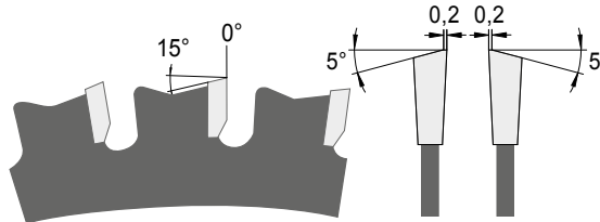
Wechselzahn mit Flachfase (W/Fa), HW
