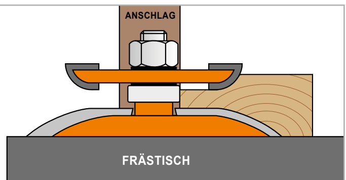
Arbeitsgang mit einem Anlaufing \varnothing 16 mm
