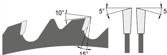
Wechselzahn (W), HW
