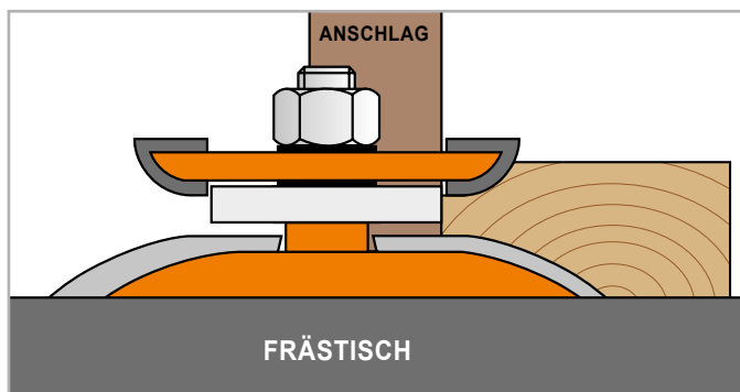
Arbeitsgang mit einem Anlaufing \varnothing 31,7 mm
